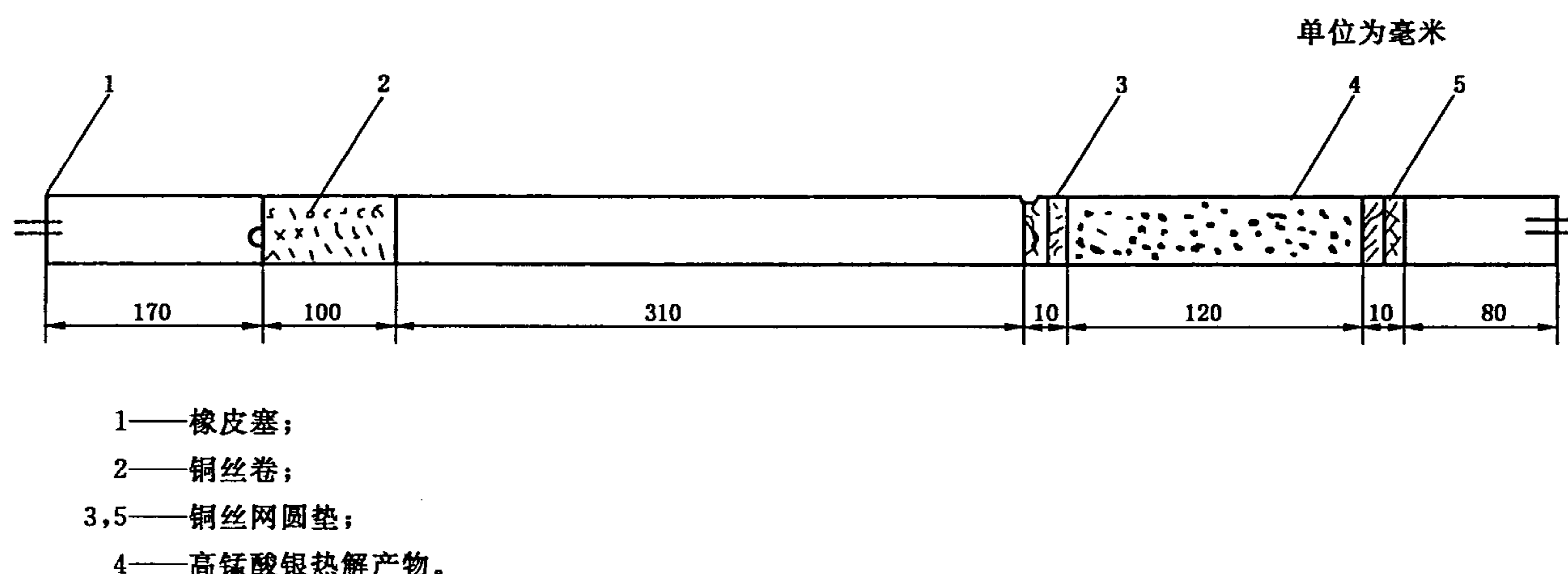
图5 二节炉燃烧管填充示意图
