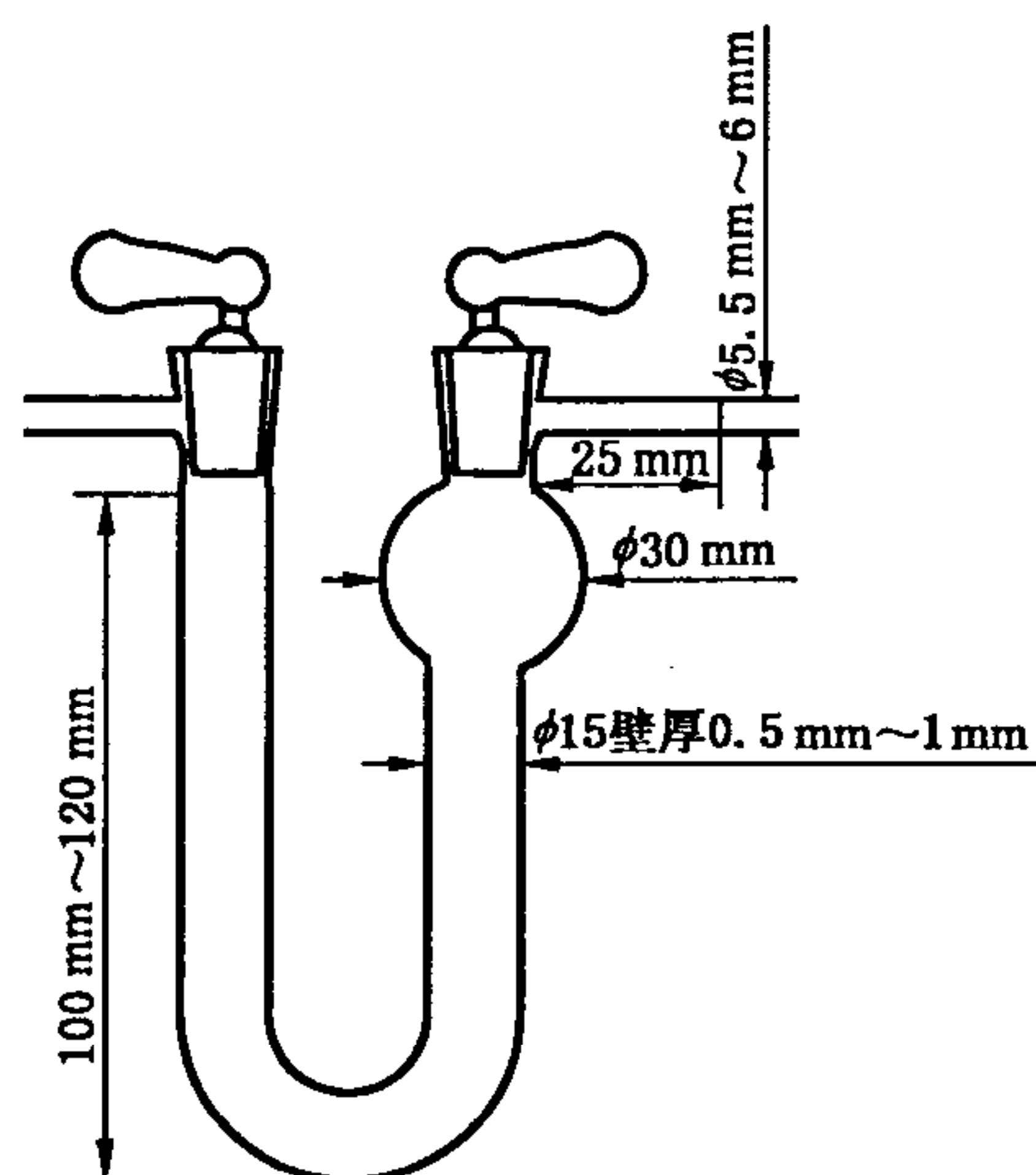
图 2 吸水 U 形管
