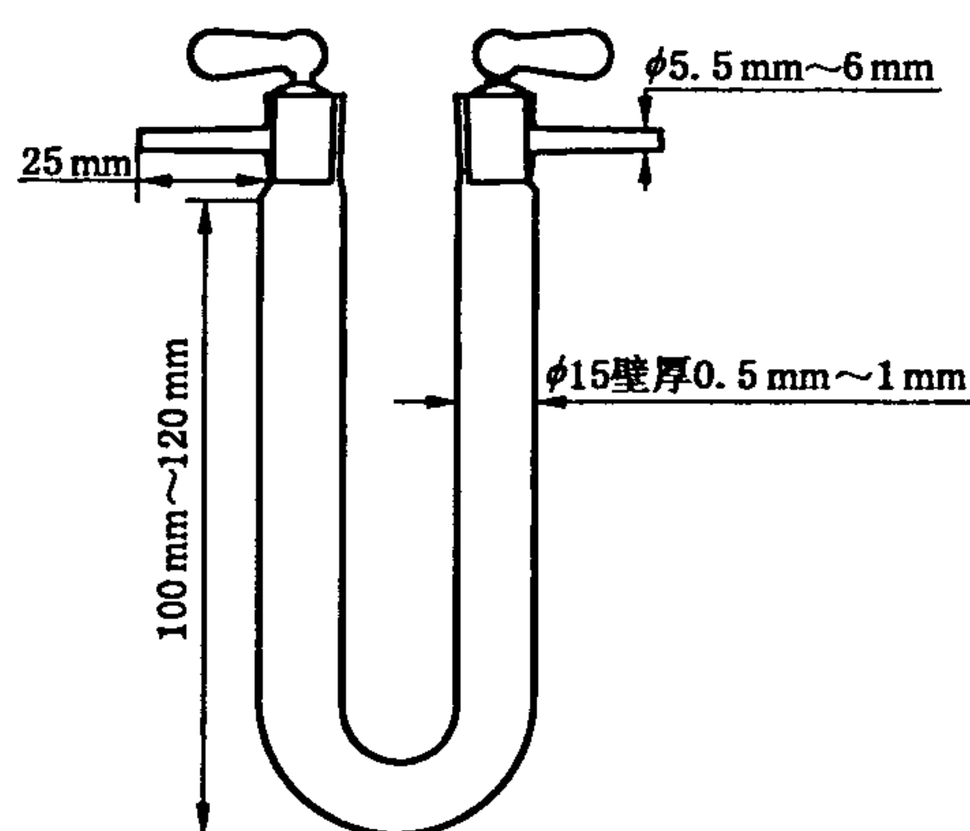
图 3 二氧化碳吸收管(或除氮 U 形管)
