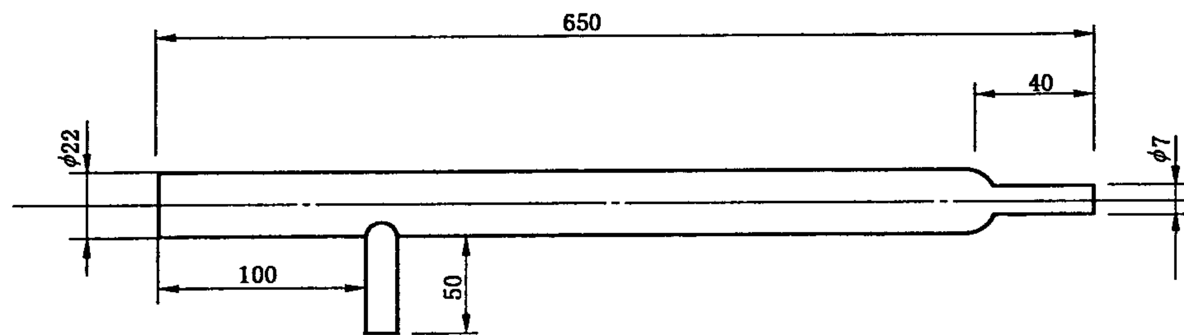
图 7 燃烧管示意图
