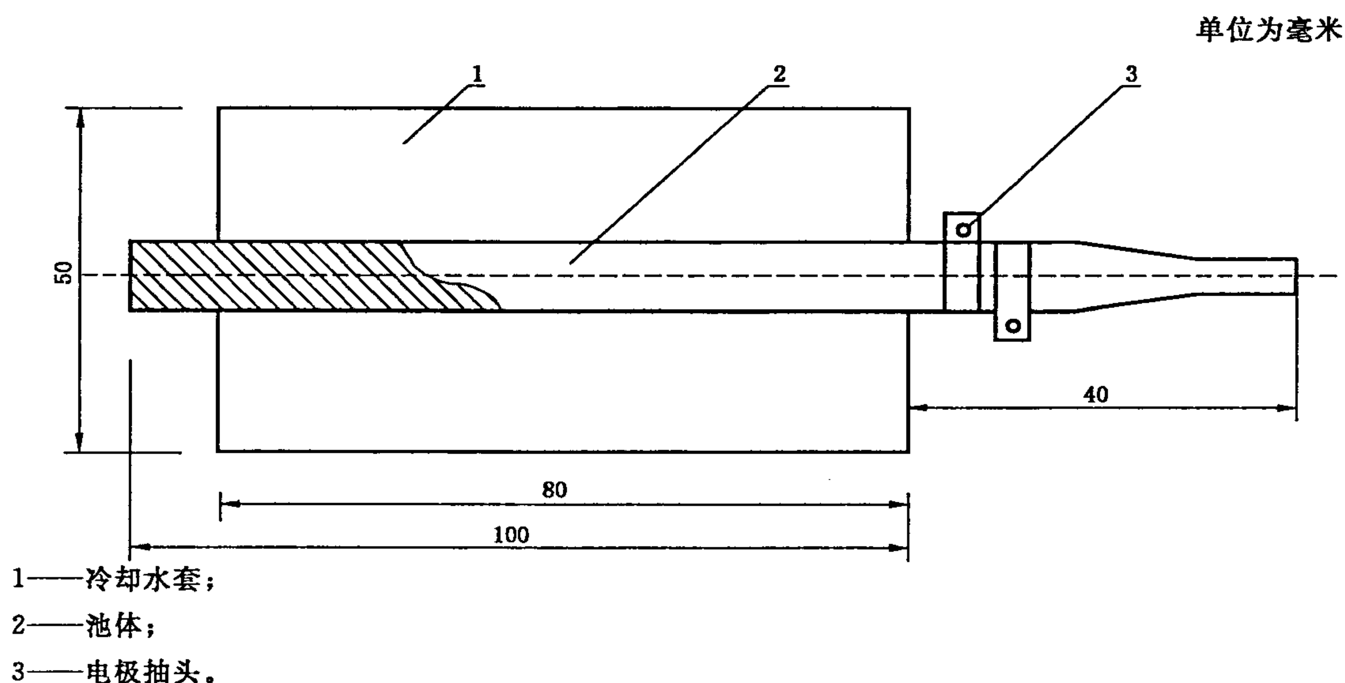
图 9 Pt-P 2 O 5 电解池示意图
