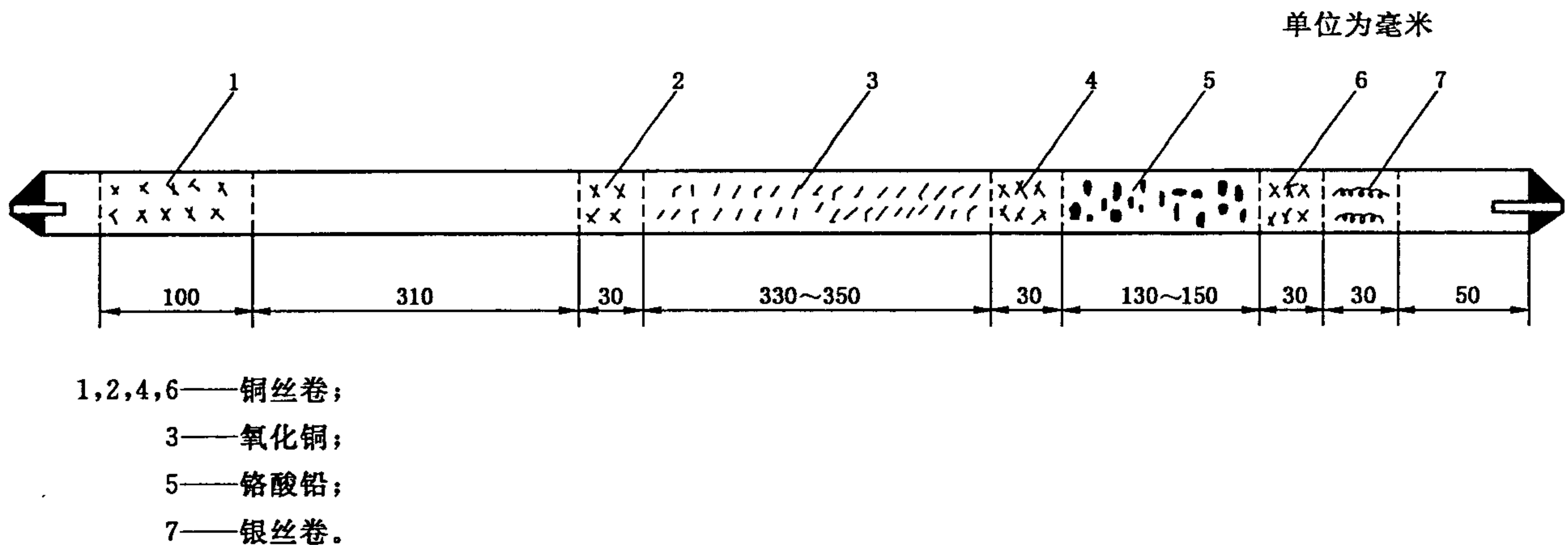
图 4 三节炉燃烧管填充示意图
